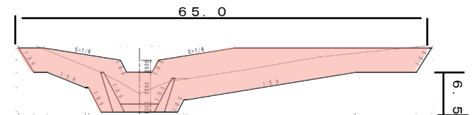
正面図
