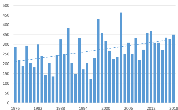
図 5-2 1時間降水量50mm以上の年間発生回数
