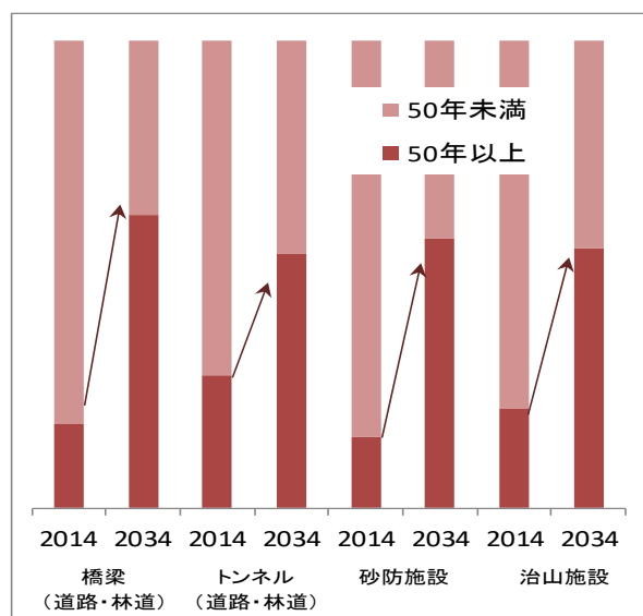
図 6-4 主な土木施設の老朽化率の見通し
