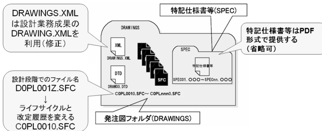
図 8-5 提供する発注図のイメージ
