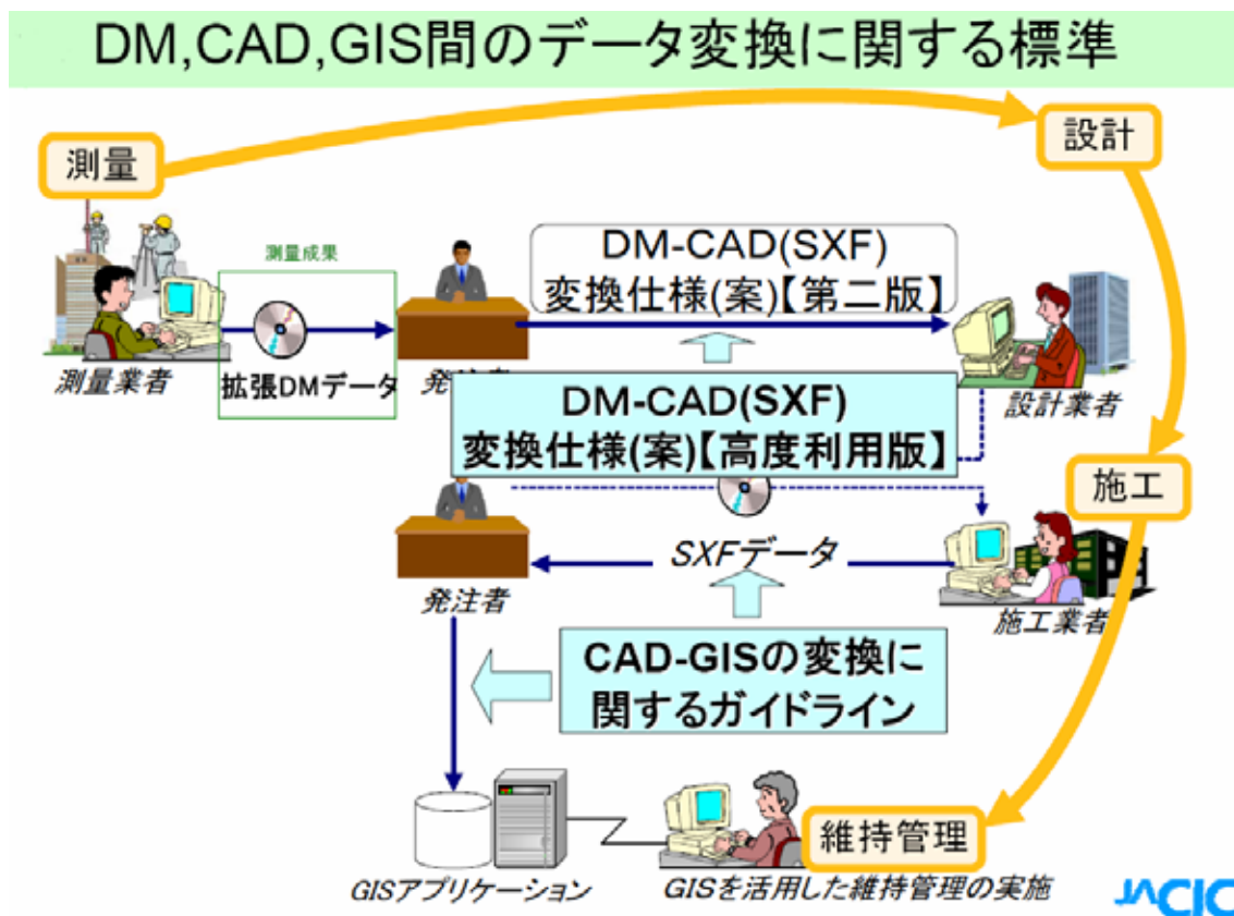
図 10-4 DM,CAD,GIS 間のデータ変換に関する標準
