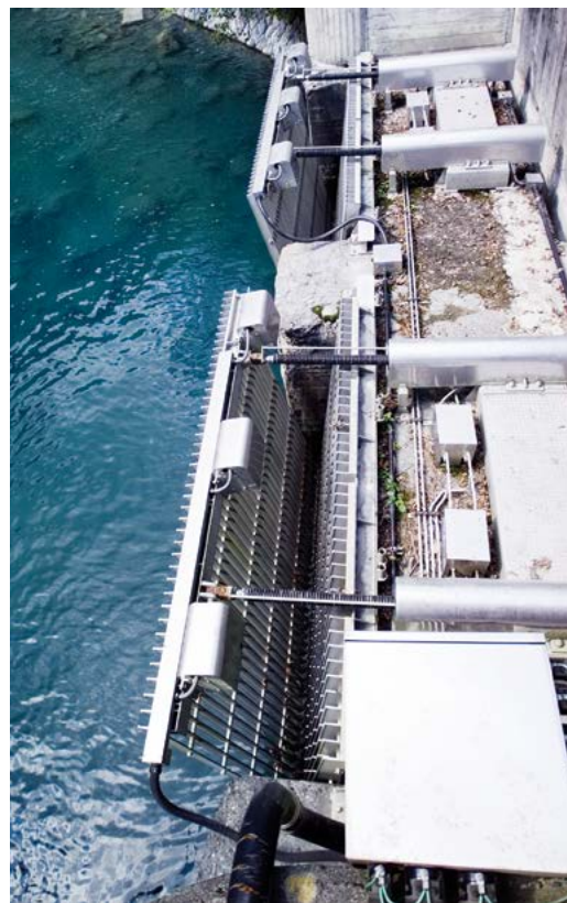
取水口可動スクリーン上部 (荒川取水口)
