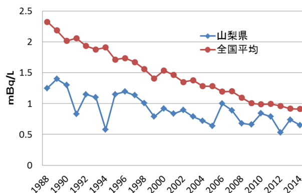
図 5 陸水中の Sr-90 経年変化
