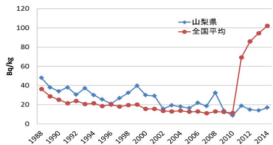
図 1 上層(0-5cm)土壌中の Cs-137 濃度経年変化
