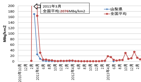
図 4 降下物中の Cs-134 経年変化
