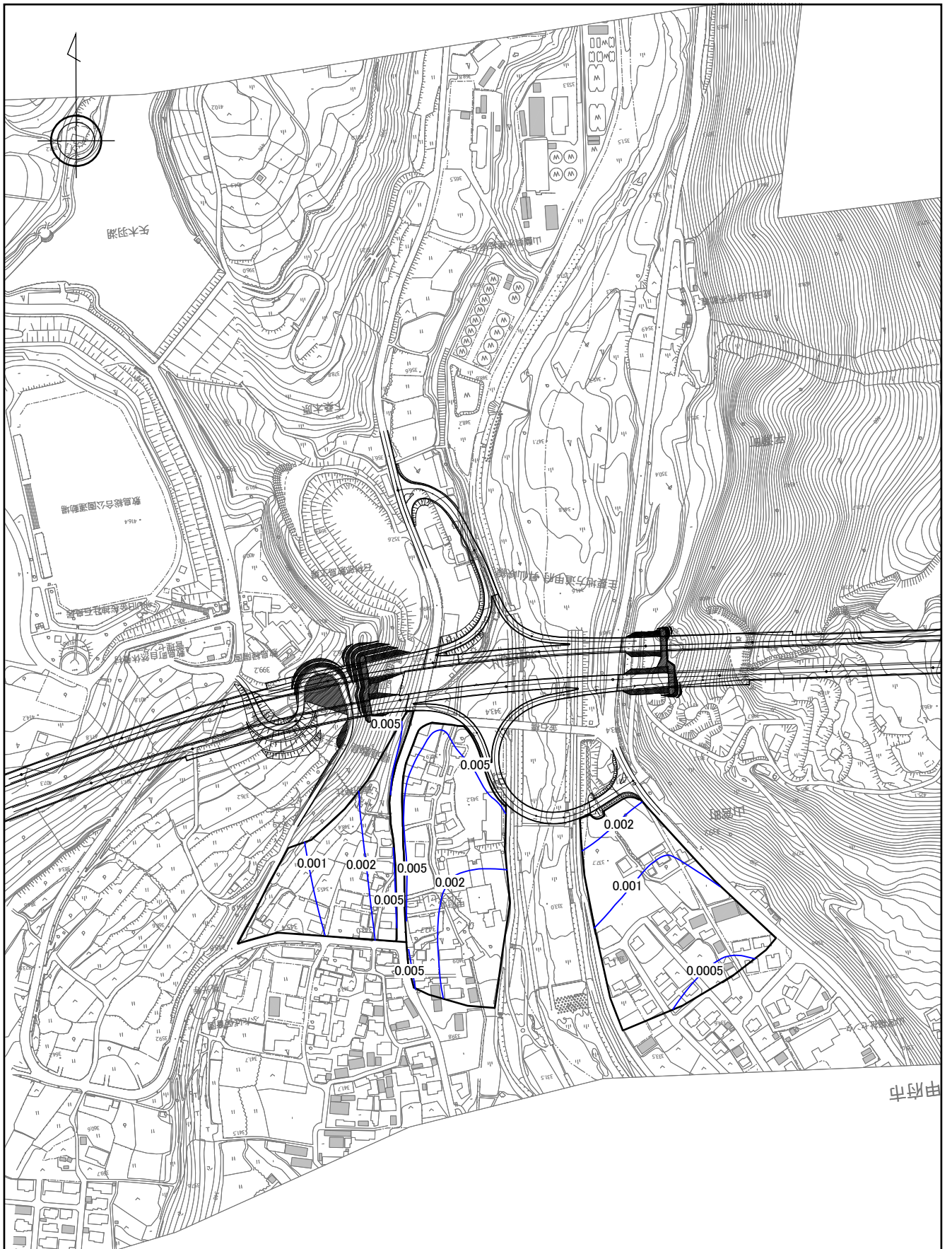
図 3-1-1 (3) 二酸化窒素等濃度線分布図 (牛久 IC 周辺)
