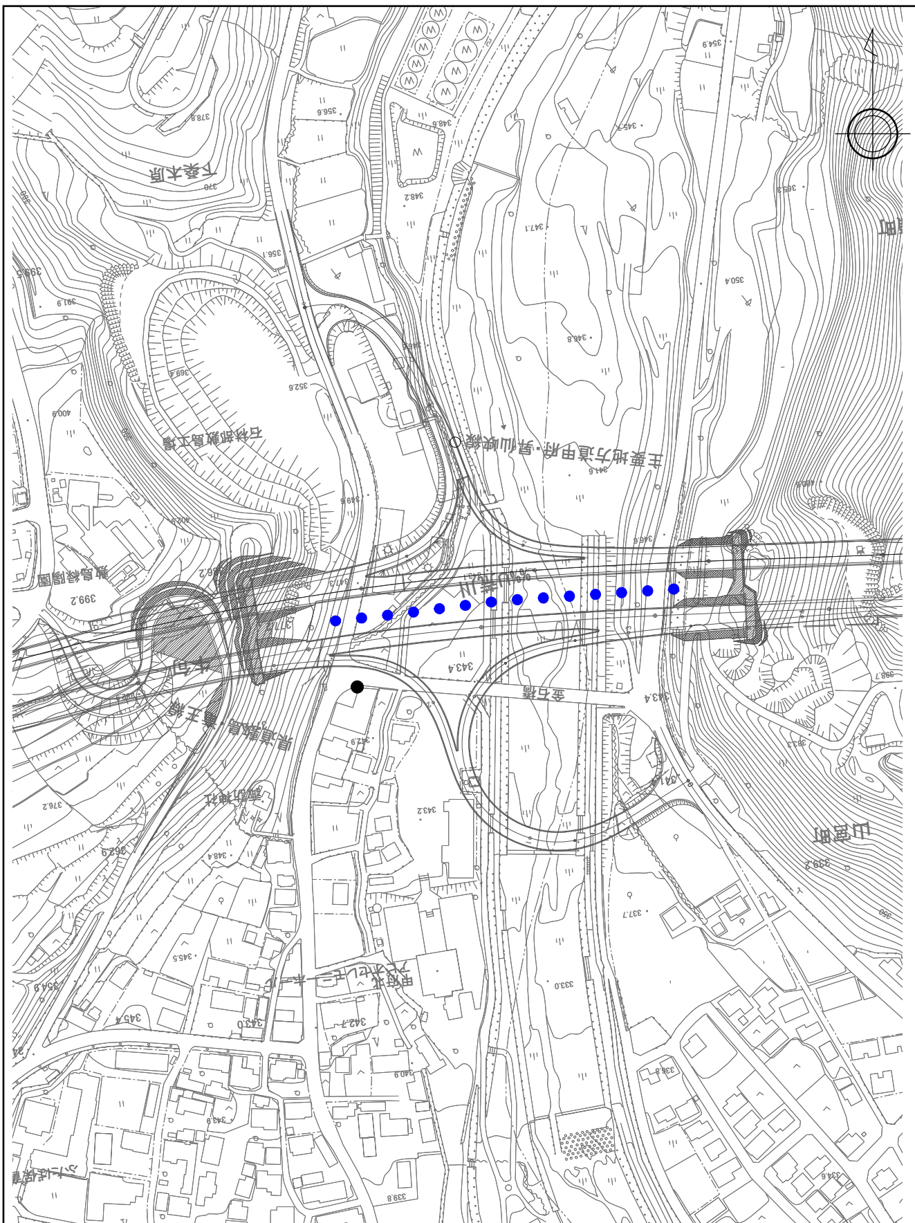
図 2-1-6(3) 甲斐市牛匂ユニット配置 (大気質)
