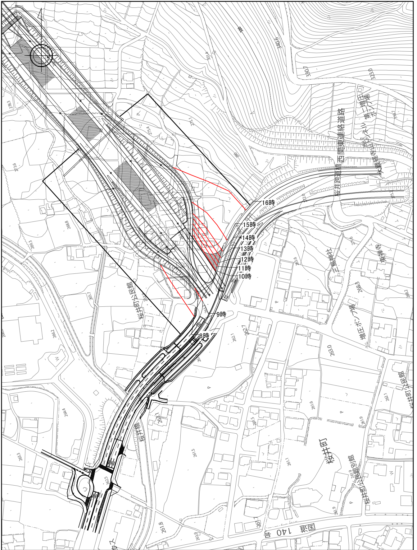
図-1-9 (1) 時刻別日影線図 (桜井 IC 周辺)
