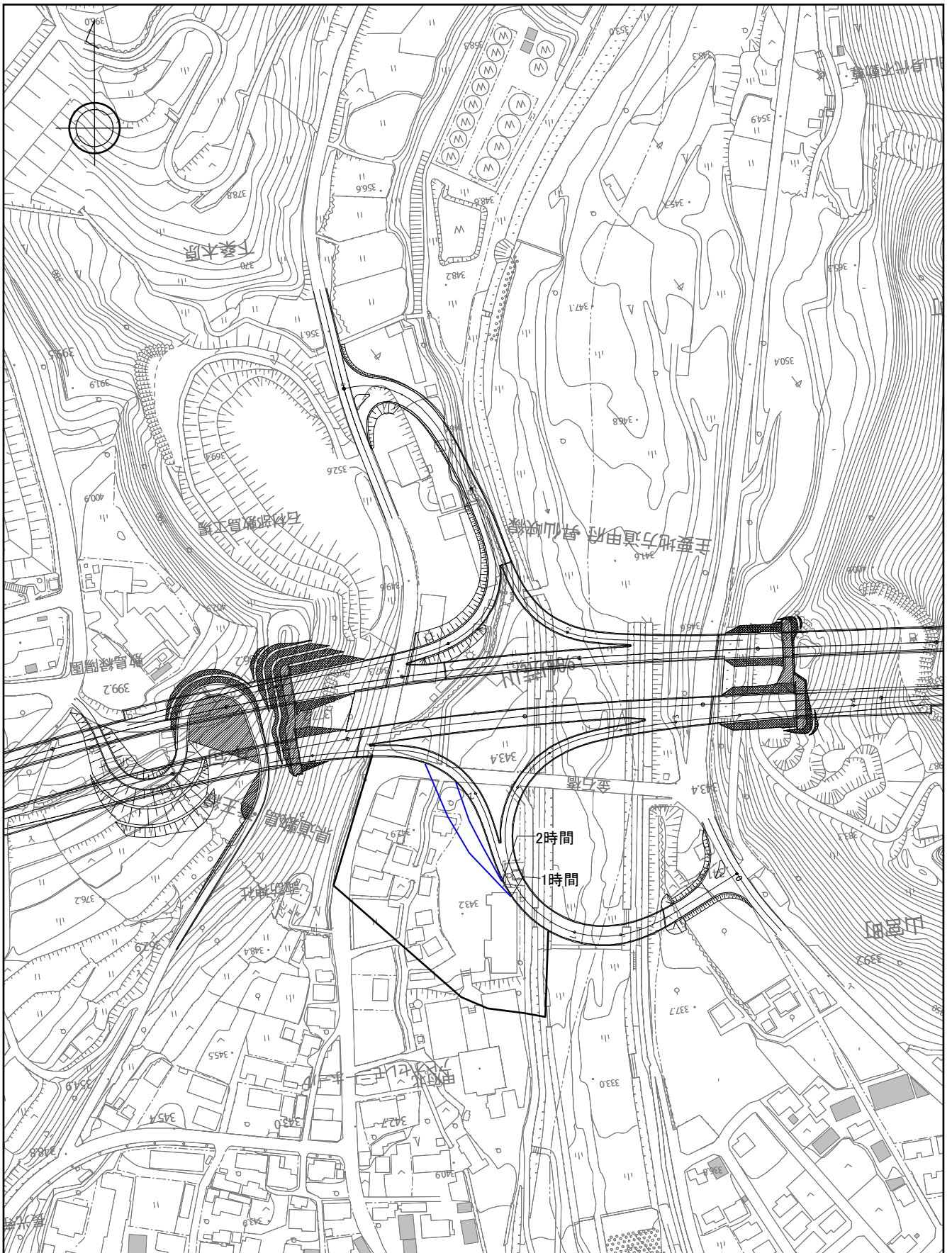
図 6-2-1 (2) 等時間日影線図 (牛久 IC 周辺)
