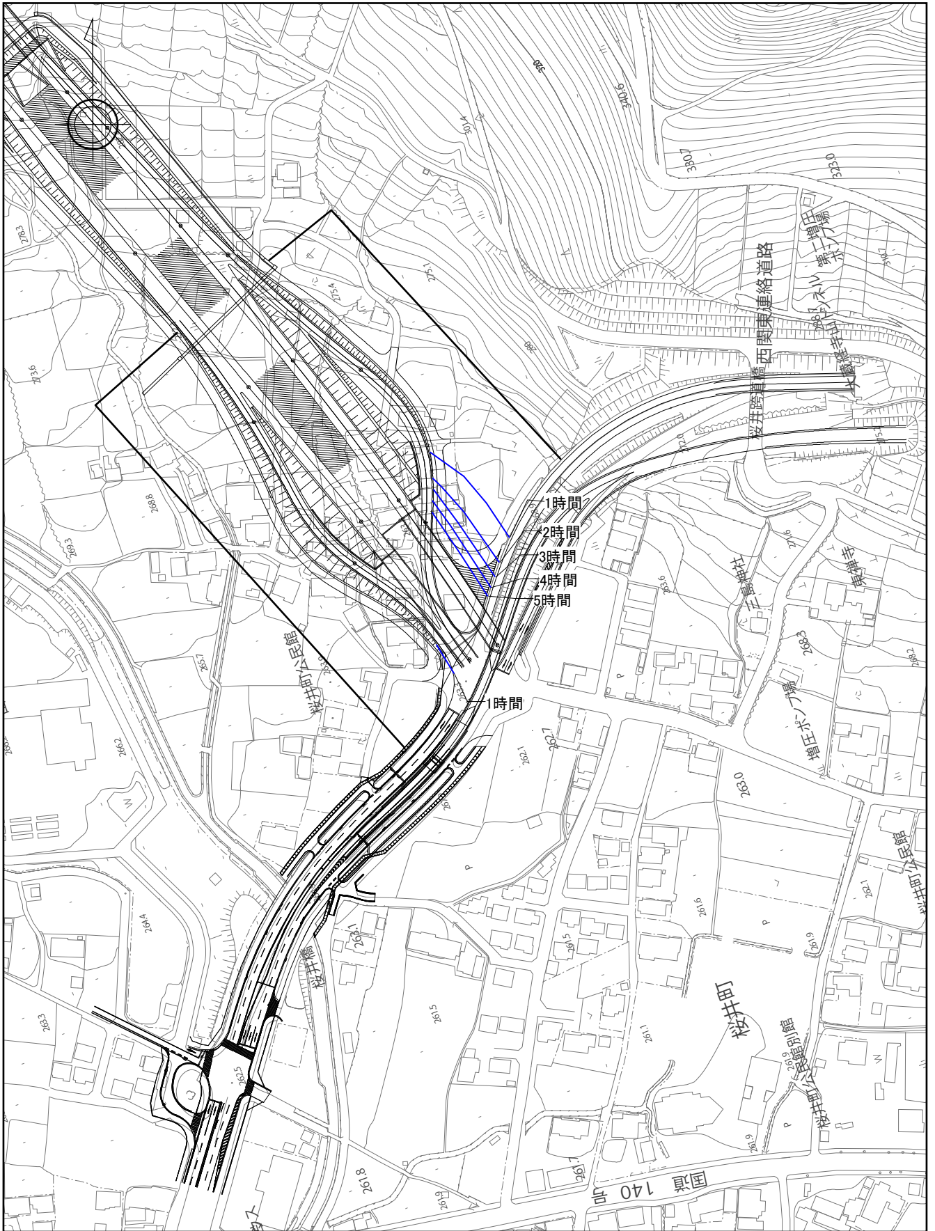
図 9-2-1 (1) 等時間日影線図 (桜井 IC 周辺)
