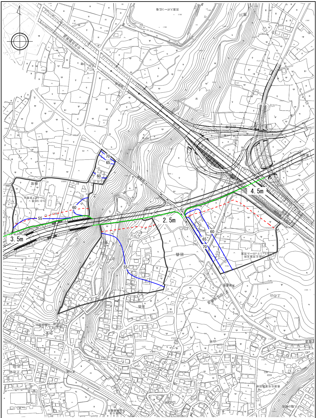
図 4-5-1 (1) 等音分布図 (岩森交差点周辺 昼間 1.2m)
