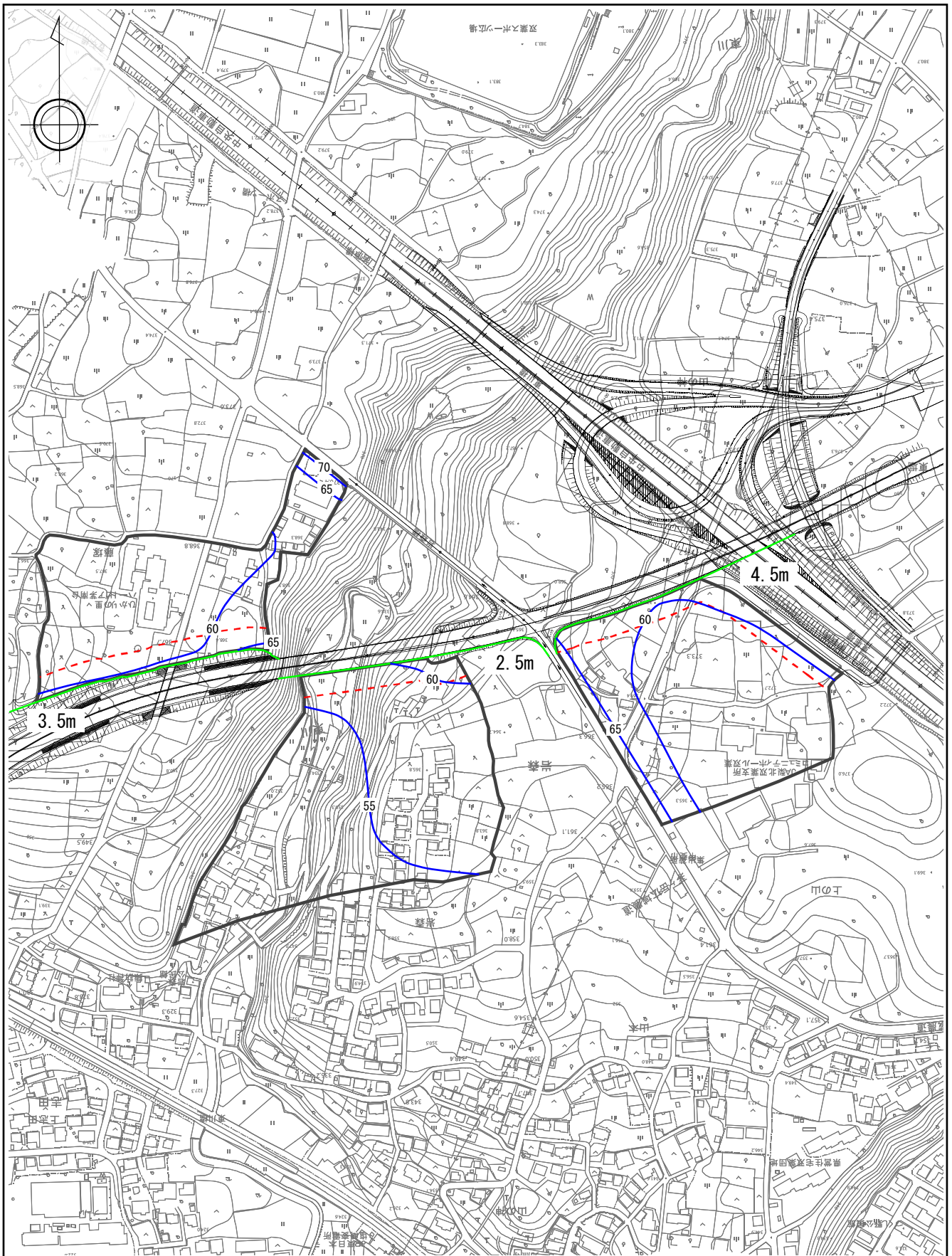
図 4-5-1 (2) 等音分布図 (岩森交差点周辺 昼間 4.2m)
