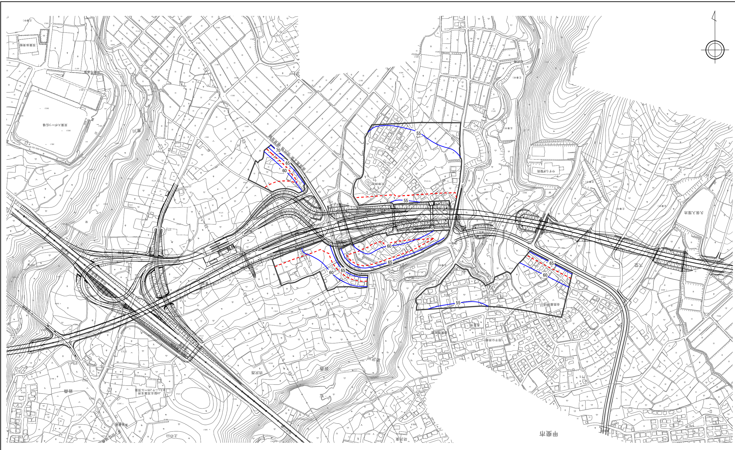
図 4-4-1 (1) 等音分布図 (甲斐 IC・JCT 周辺 昼間 1.2m)
