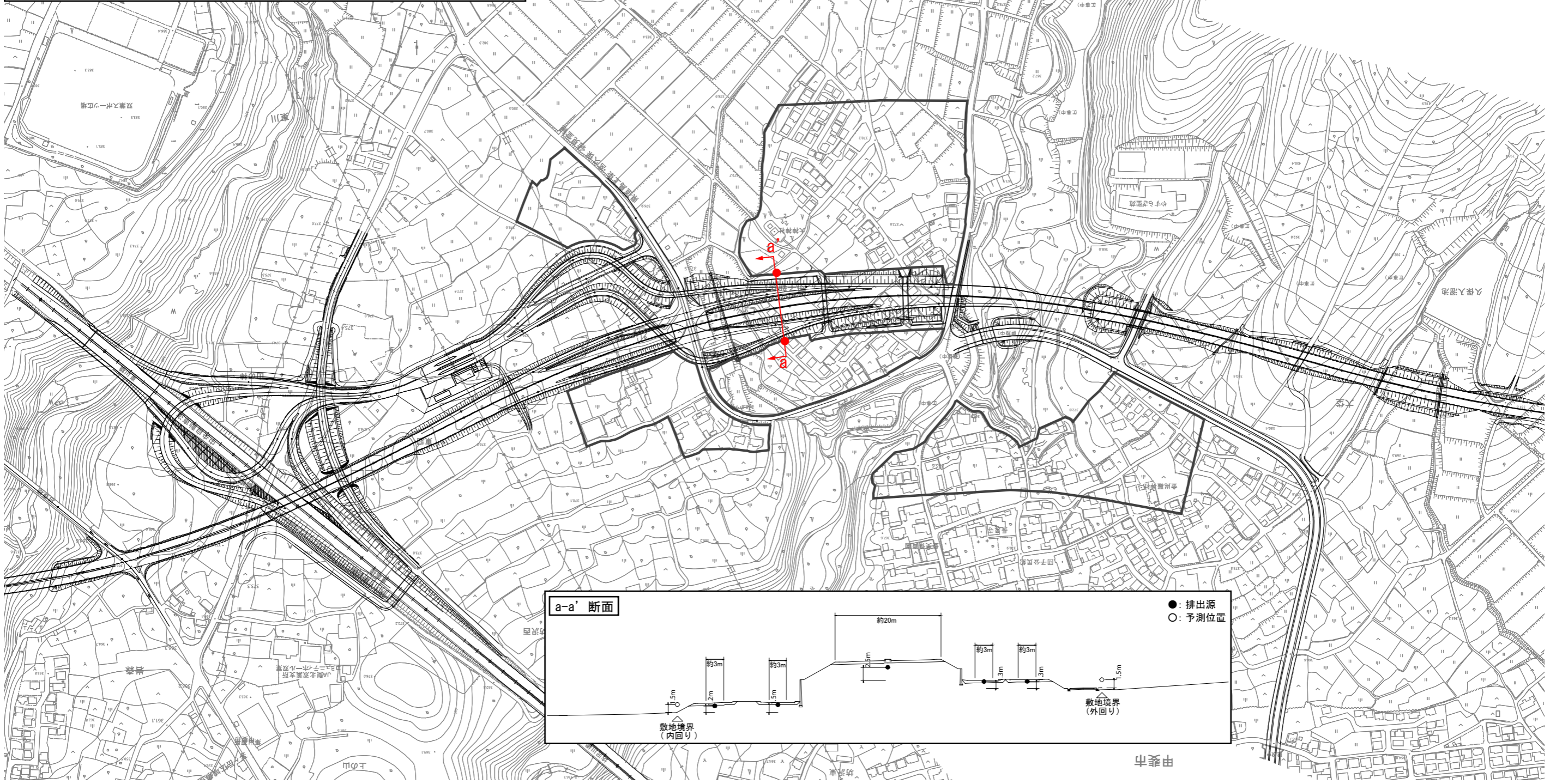
図 8-1-8 (4) 予測範囲図 (甲斐 IC・JCT 周辺)
