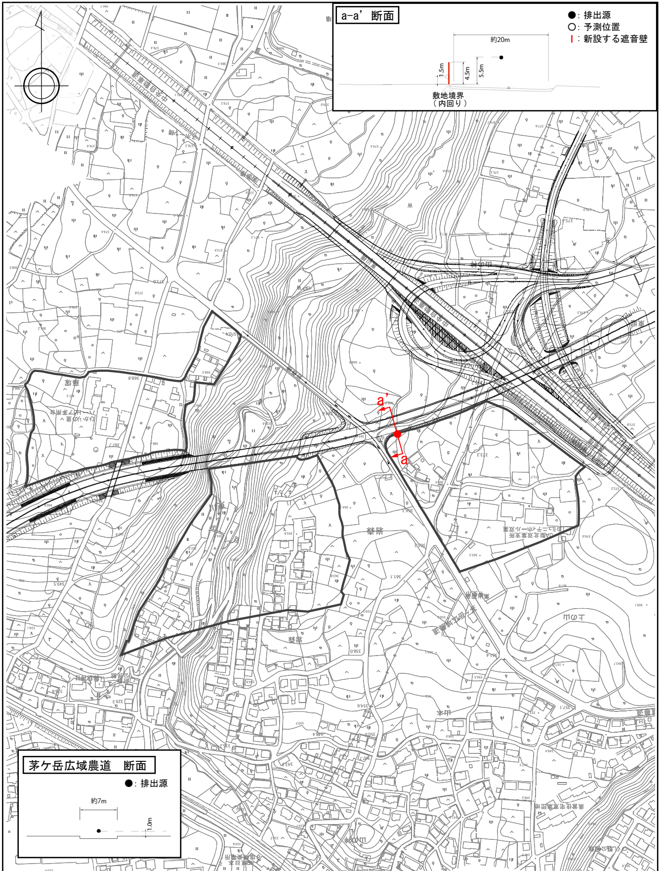
図 8-1-8 (5) 予測範囲図 (岩森交差点周辺)
