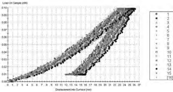
図11 GZO1における荷重—押し込み深さ曲線
