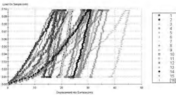
図12 GZO3における荷重—押し込み深さ曲線
