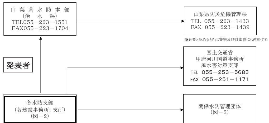
図ー1-1 相模川水系各河川の水防警報連絡系統図
