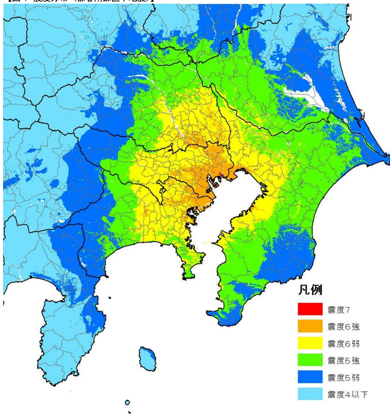
【図1 震度分布（都心南部直下地震）】
