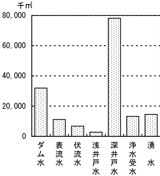
上水道・簡易水道における 水源別取水量
