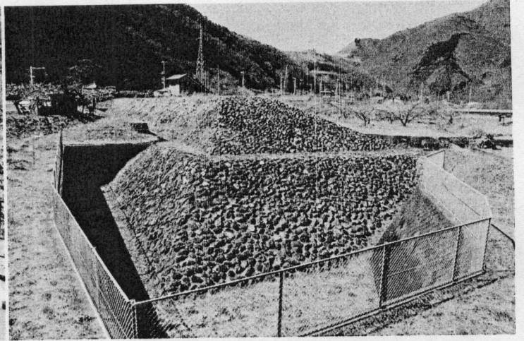
石積出三番堤
