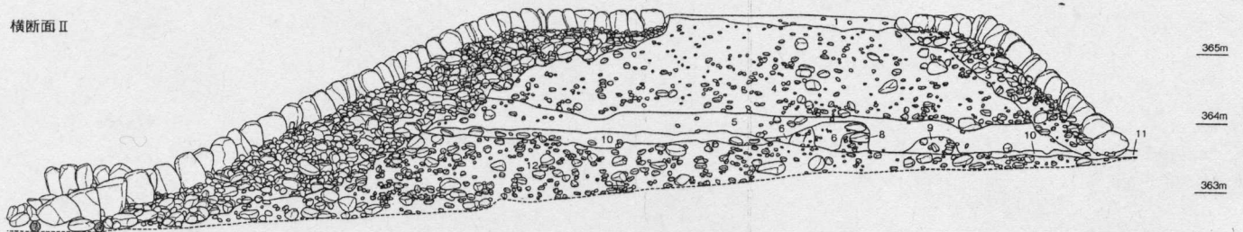
塩川 塩川下河原堤防
