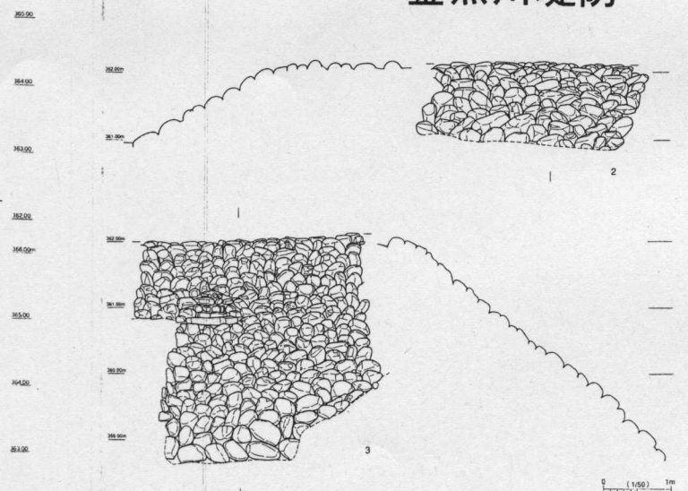
釜無川 西表堤防
