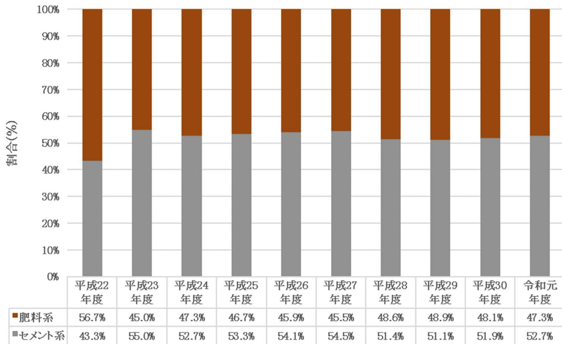
【図5-4 汚泥処理先別推移】
