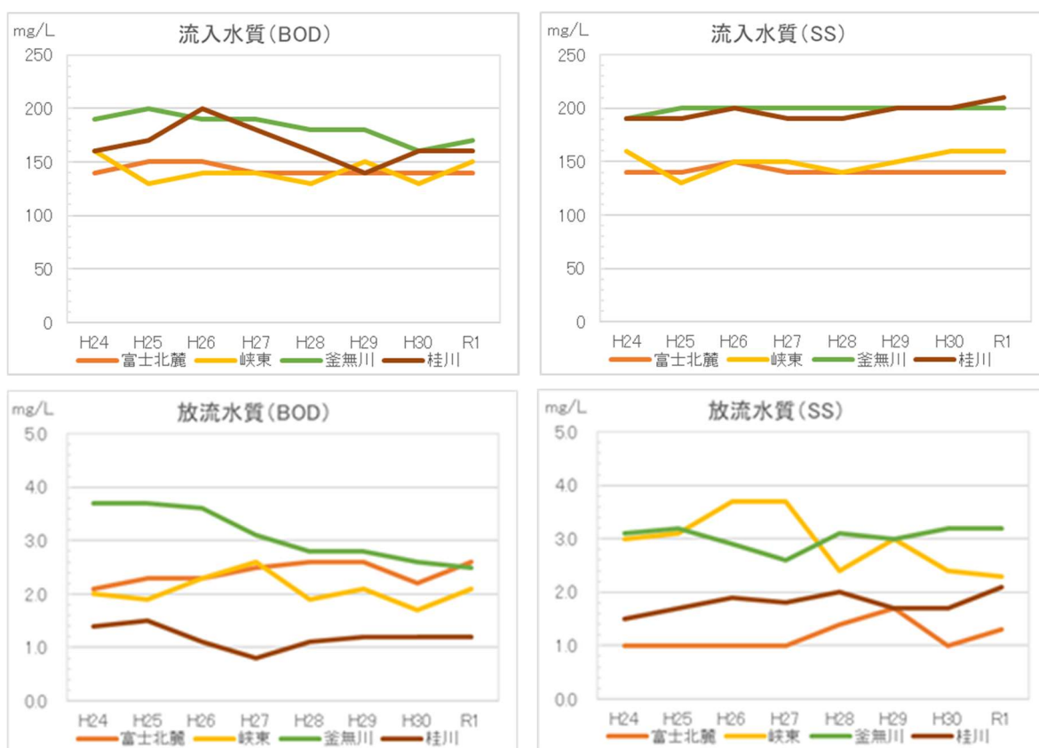
【図5-1 流入水質及び放流水質の経年変化（年平均値）】
