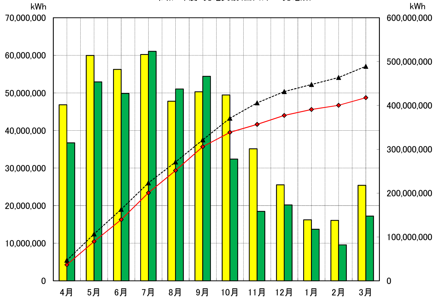
月別目標・実績供給電力量 令和3年度 発電実績(西山外26発電所)
