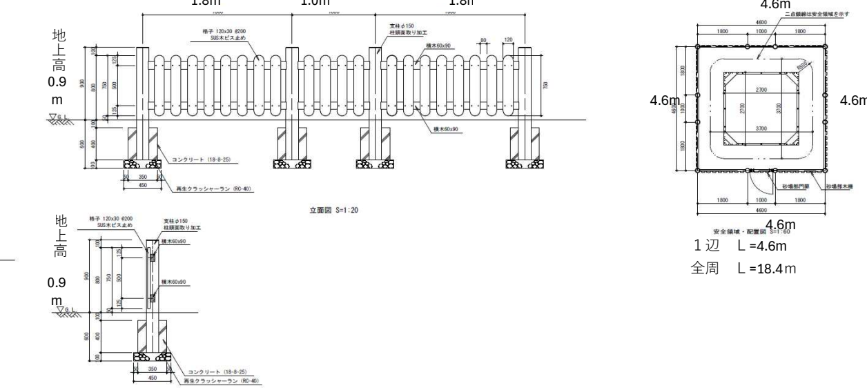
④砂場外周柵・門扉更新工
