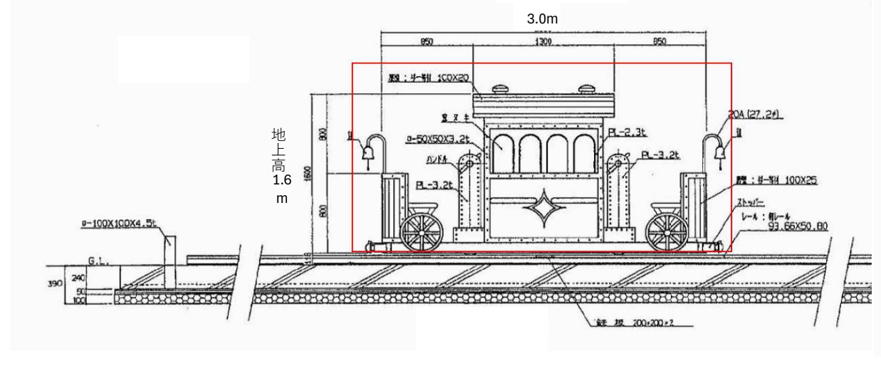
⑤鉄道撤去工（手漕ぎ機関車）※赤枠内を撤去
