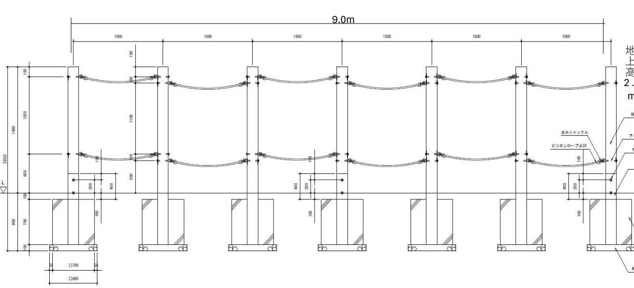
③ロープ渡り更新工
