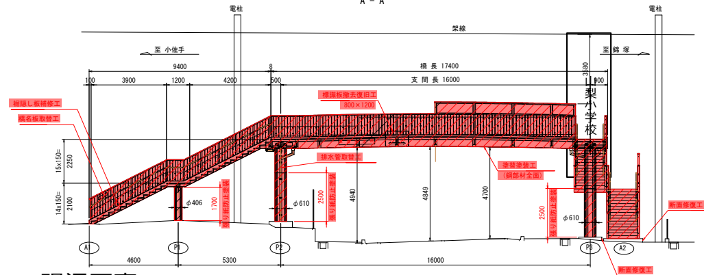
側面図 S=1/100
