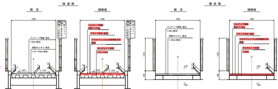
上部工横断面図 S=1/20
