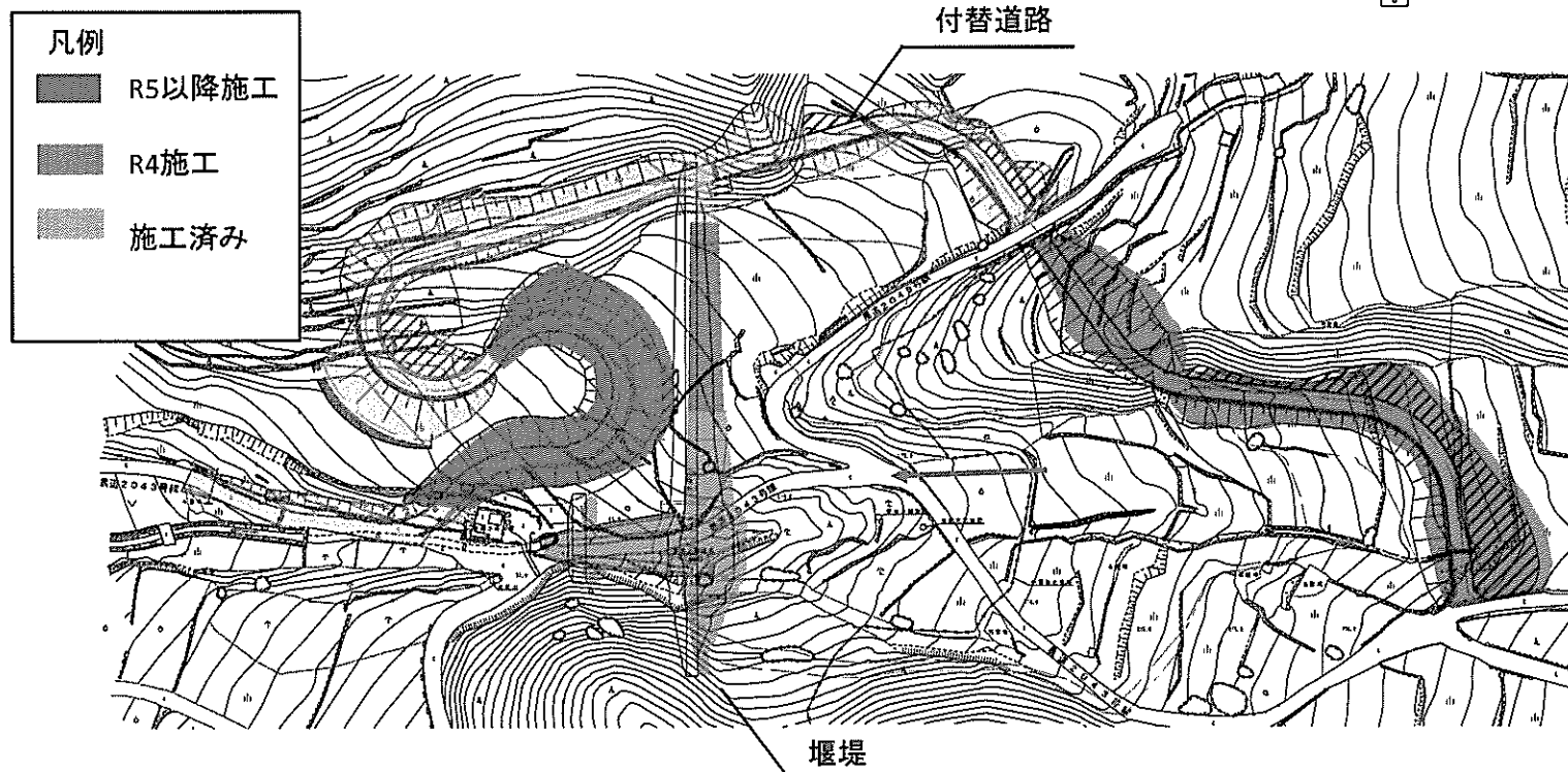
平面図
