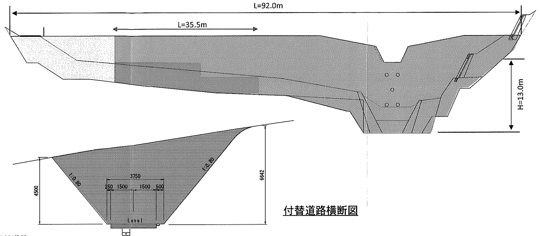
堰堤正面図
