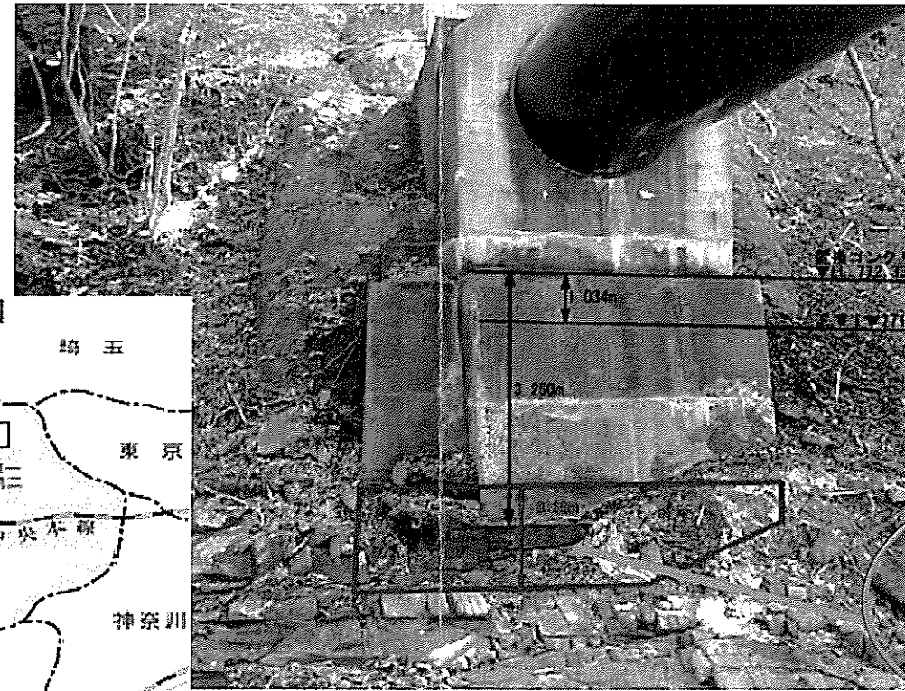
写真1：施工箇所
