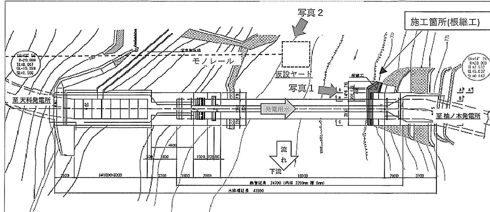
平面図
