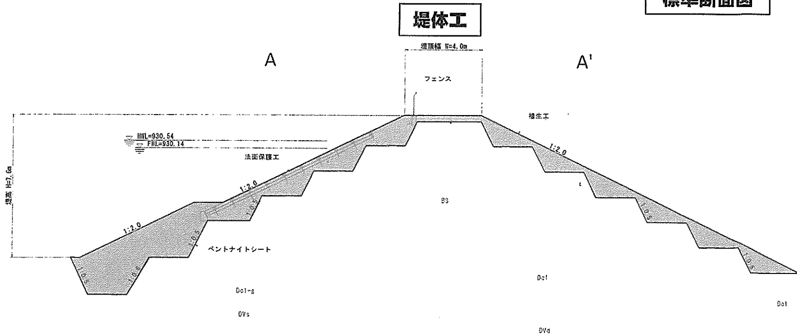
標準断面図
