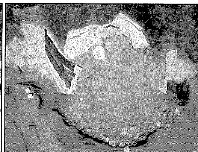
斜面の再崩壊状況(令和3年7月21日)
