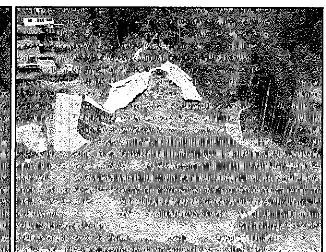
抑え盛土による応急復旧状況
