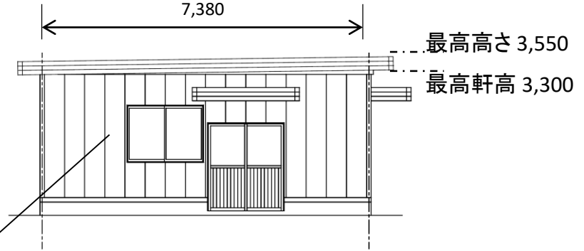
南側立面図
