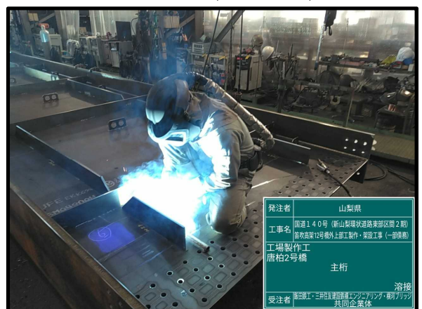
施工状況(橋桁溶接)
