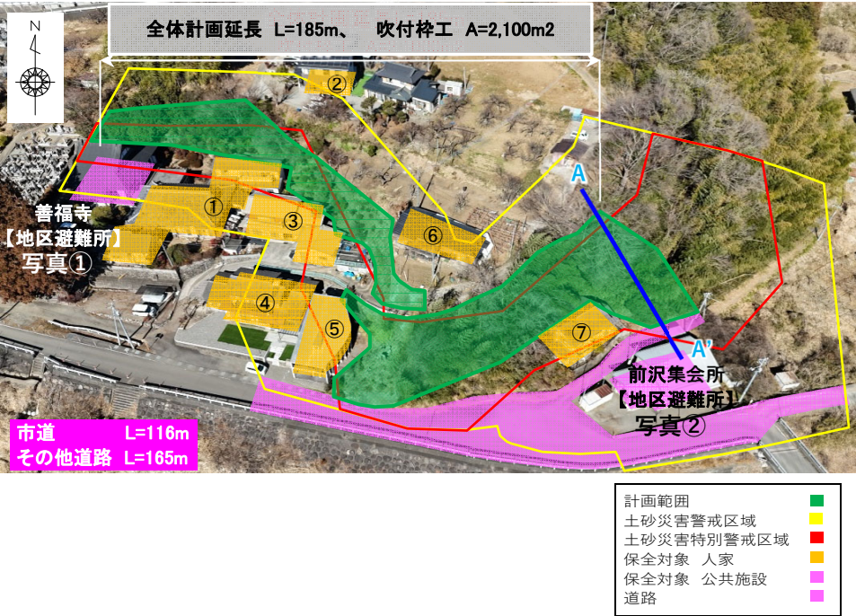
【斜面鳥瞰図】
