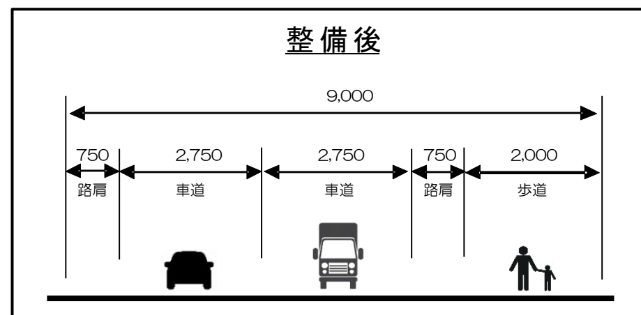
標準断面図
