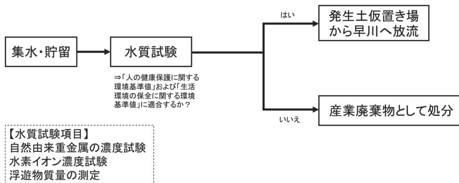
図 4-1-1-2 排水処理のフロー
