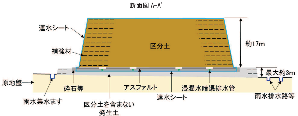
図 2-3(2) 中洲地区（その 2）発生土仮置き場計画地における盛土計画
