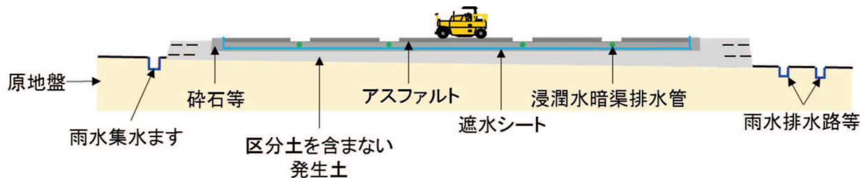
図 2-5(1) 主な施工手順（アスファルト舗装施工）
