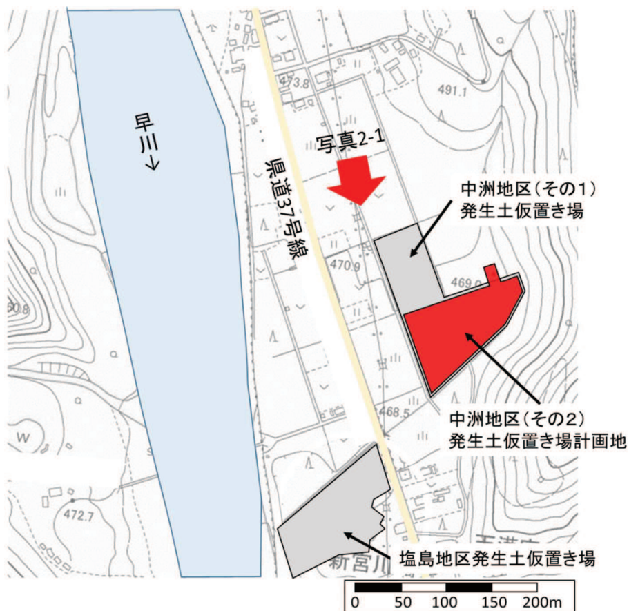
図 2-2 中洲地区（その 2）発生土仮置き場計画地平面図
