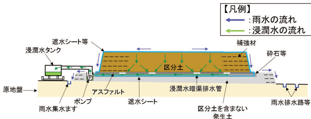
図 2-4 排水計画概要図
