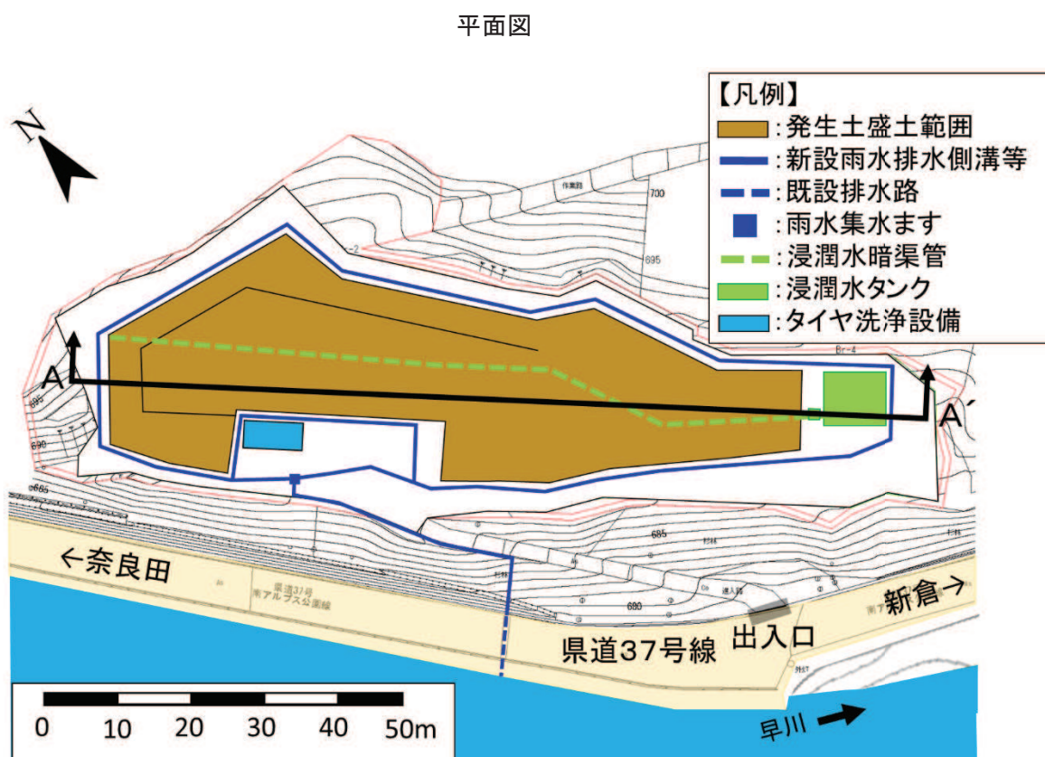
図 2-3(1) 湯島地区（田島）発生土仮置き場における盛土計画
