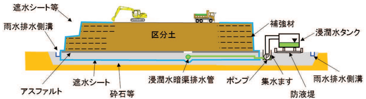
図 2-5 (4) 主な施工手順（区分土搬出）
