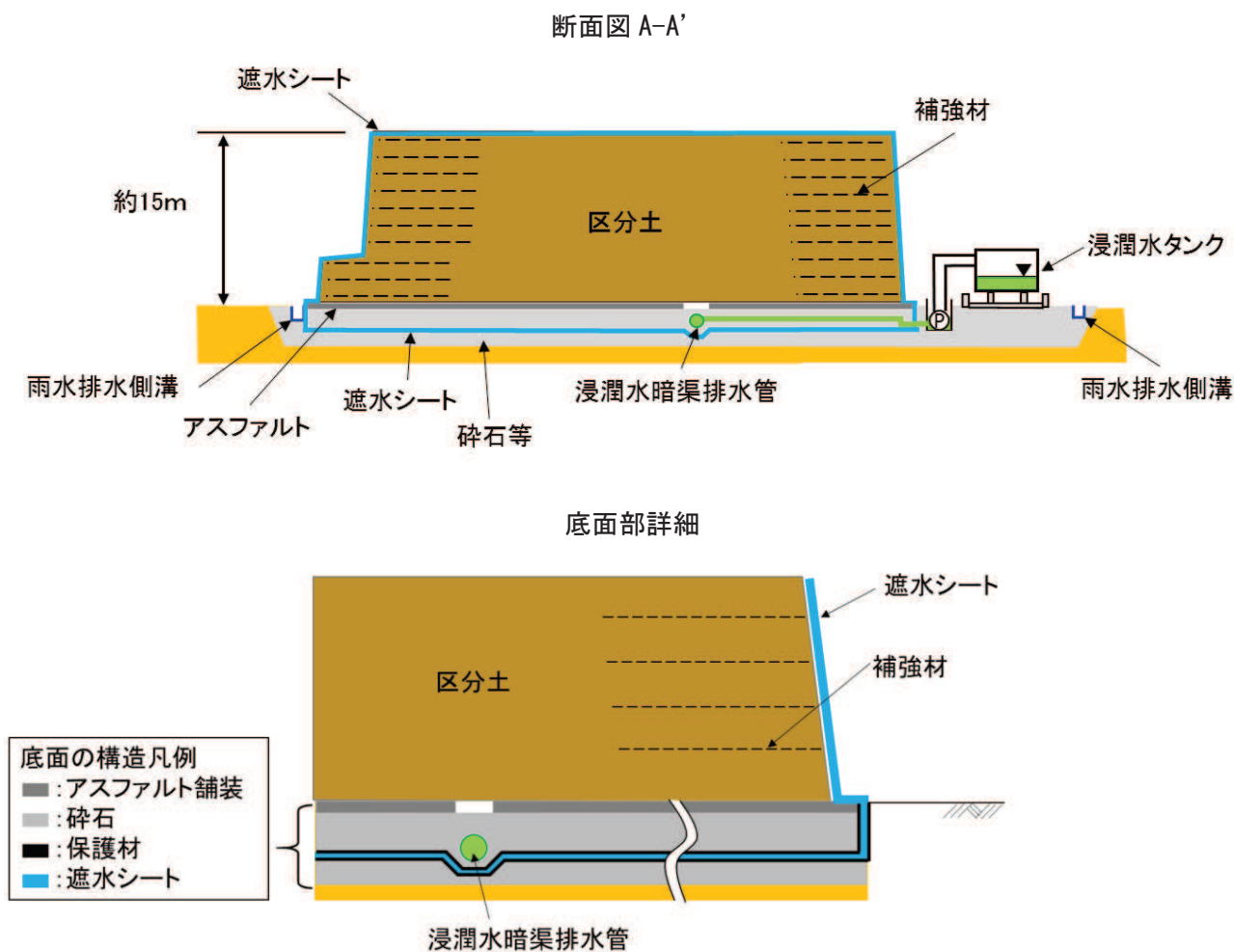
図 2-3(2) 湯島地区（田島）発生土仮置き場における盛土計画
