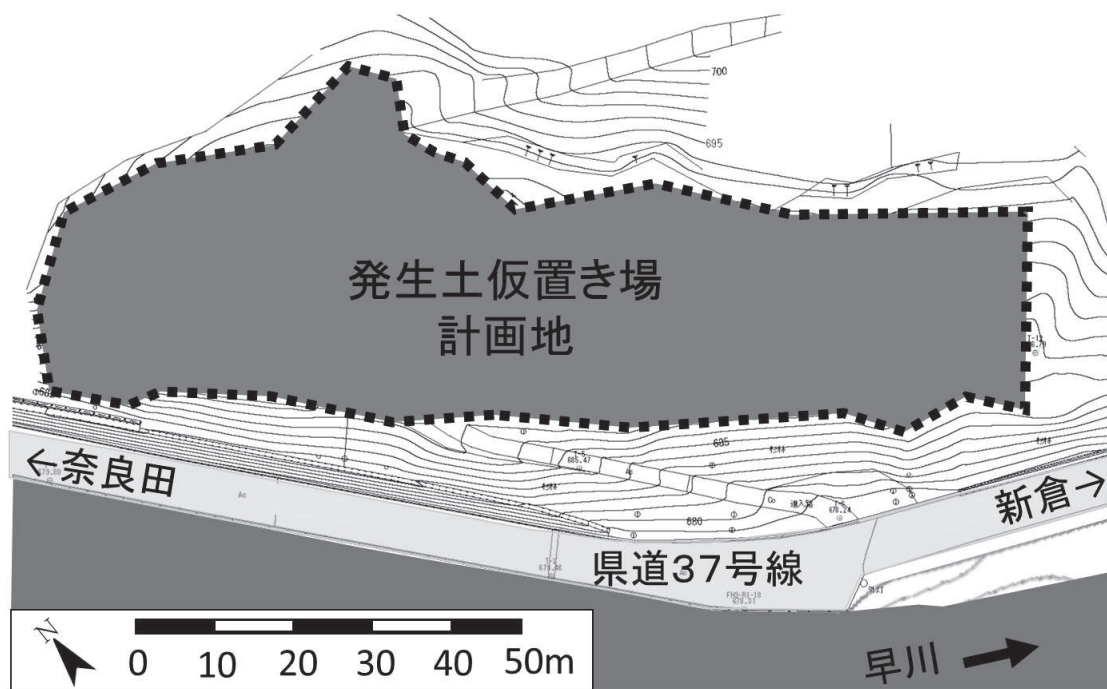
図 2-2 湯島地区（田島）発生土仮置き場計画地平面図（現況）
