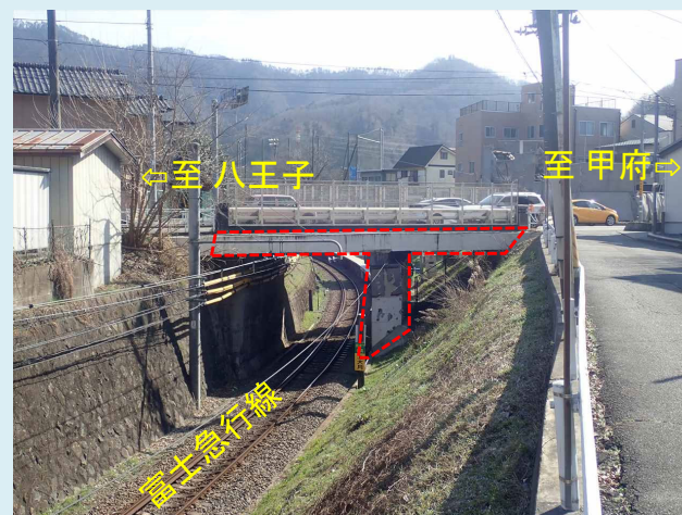
てんのう ② 天王橋 【橋梁補修】主桁補修、橋脚補修等
