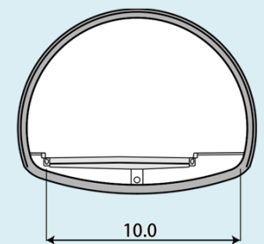
＜新設トンネル断面＞
