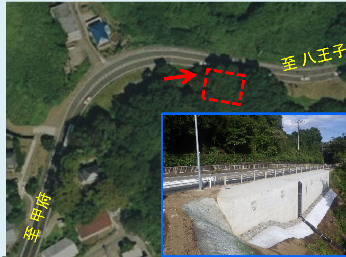
② 【R3補正対策工事】山梨県上野原市四方津地先 【防災対策】場所打法砕工等→R5.10完成
