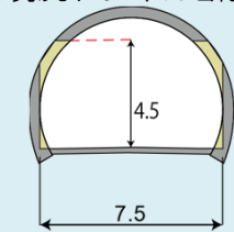
＜現況トンネル断面＞
