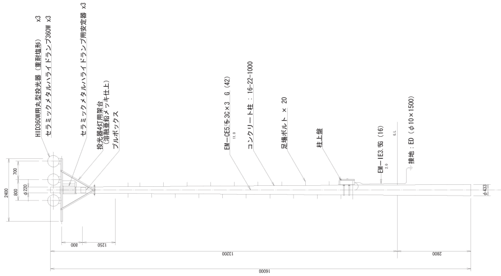
照明塔姿図 S=1:50
