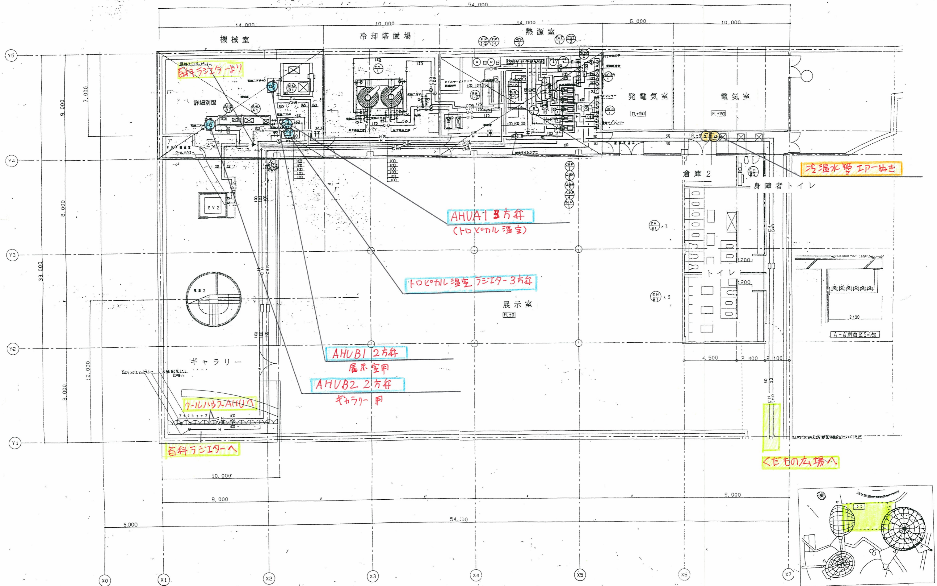
くだもの百科 BIF 配管 平面図 S=1/100
